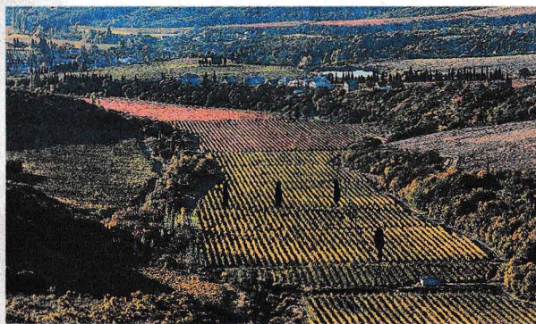
Рис. 120. Аграрный ландшафт
