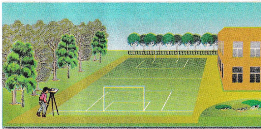
Рис. 28. Съёмка местности
