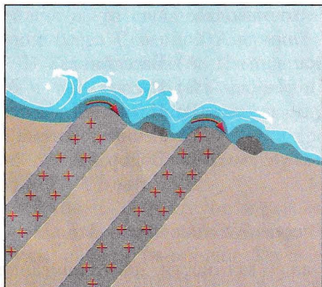
Рис. 74. Схема порогов
