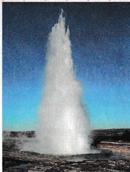
Рис. 49. Гейзер
