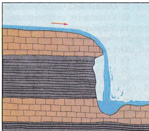
Рис. 75. Схема водопада
