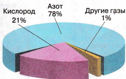
Рис. 83. Состав воздуха
