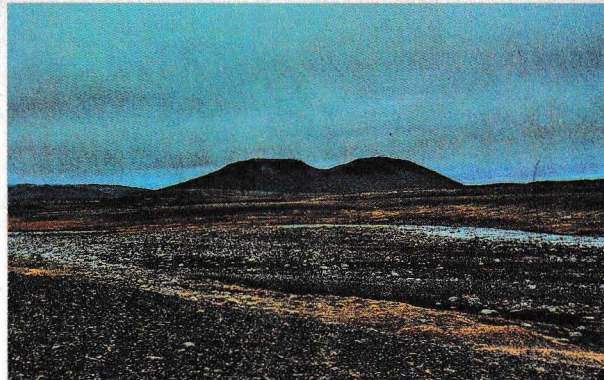
Рис. 119. Арктическая пустыня
