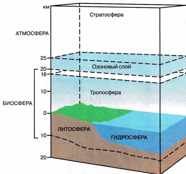
Рис. 103. Границы биосферы
