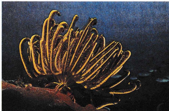
Рис. 63. Морская лилия
