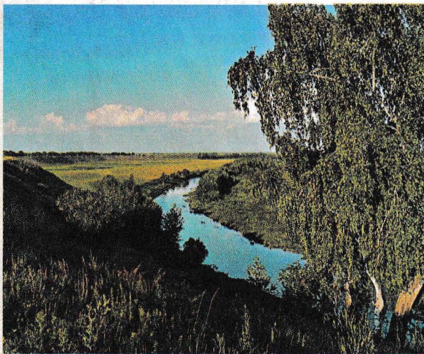
Рис. 53. Восточно-Европейская равнина
